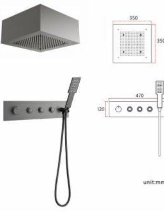
11AH3+1S142W-Q 3 功能恒温套装（枪灰） Three -features thermostatic set (Gunmetal) 雨淋、喷雾、手持 Rain shower, atomizing, hand 单位 Unit： mm
