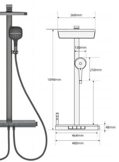
MZ1090464-Q 恒温配套（枪灰） Temperature control set (Gunmetal) 淋浴、手持、喷枪 Shower, hand, Spray gun
