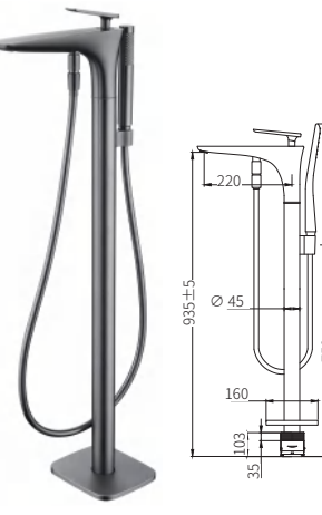
LD001-Q 暗装落地浴缸龙头（枪灰） Concealed floor-to-ceiling bathtub mixer (Gunmetal) (可定制明装)
