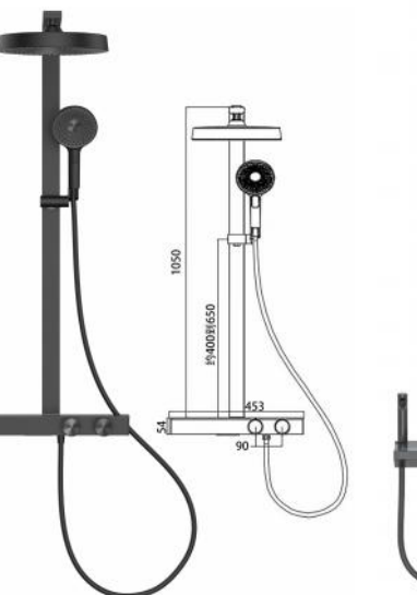
MZ940450-Q 调温配套（枪灰） Thermoregulation control set (Gunmetal) 淋浴、手持 Shower, hand
