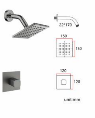
49T1B06-Q 单功能调温配套（枪灰） Single function thermoregulation set (Gunmetal) 淋浴 Shower 单位 Unit: mm
