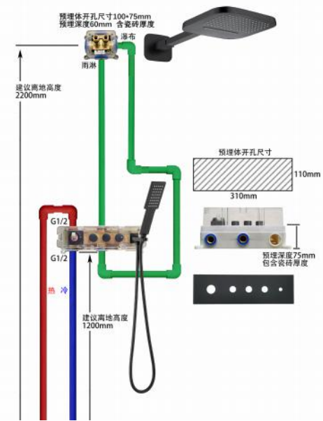
05AH3+1B152-Q 3 功能恒温套装（枪灰） Three-function thermostatic set (Gunmetal) 双瀑布、雨淋、手持 Double waterfall, rain , hand 单位 Unit: mm
