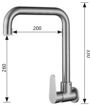
GCP320-S 304 不锈钢单冷厨房龙头（拉丝） 304 stainless steel kitchen mixer (Brushed) 单位 Unit: mm
