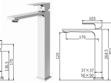
TS26850 铜面盆龙头（铬色） Brass basin mixer (Chrome) 单位 Unit: mm
