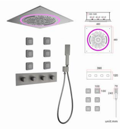
99T4B192LJ4-Q 4 功能 LED 调温套装（枪灰） Four -features LED thermoregulation set (Gunmetal) 雨淋、双瀑布、背喷、手持 Rain shower, double waterfall,back spray, hand 单位 Unit: mm
