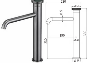
TS33042-Q 铜面盆龙头（枪灰） Brass basin mixer (Gunmetal) 单位 Unit: mm
