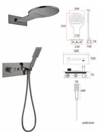
05AH3+1B122-Q 3 功能恒温套装（枪灰） Three-function thermostatic set (Gunmetal) 单瀑布、雨淋、手持 Single waterfall, rain, hand 单位 Unit: mm
