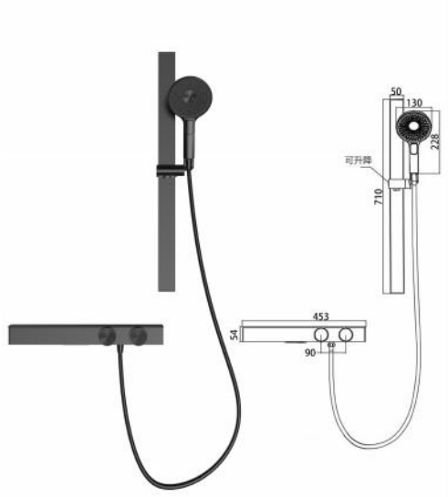
MZ450S-Q 调温配套（枪灰） Thermoregulation control set (Gunmetal) 淋浴、手持 Shower, hand
