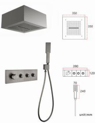
13AH3S142-Q 3 功能恒温套装（枪灰） Three -features thermostatic set (Gunmetal) 雨淋、瀑布、手持 Rain shower, waterfall, hand 单位 Unit： mm
