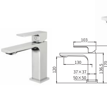
TX13650 铜面盆龙头（铬色） Brass basin mixer (Chrome) 单位 Unit: mm
