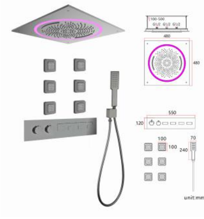
14AH4S192LJ4-Q 4 功能 LED 恒温套装（枪灰） Four -features LED thermostatic set (Gunmetal) 雨淋、双瀑布、背喷、手持 Rain shower, double waterfall, back spray, hand 单位 Unit: mm
