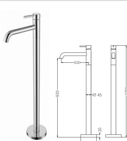
LZR01 明装装落地浴缸龙头（铬色） Floor-to-ceiling bathtub mixer (Chrome)
