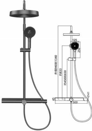
MZ940500-Q 调温配套（枪灰） Thermoregulation control set (Gunmetal) 淋浴、手持 Shower, hand
