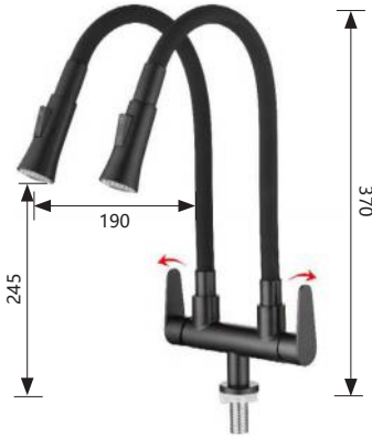
GCP370-2H 304 不锈钢单冷厨房龙头（黑色） 304 stainless steel kitchen mixer (Black) 单位 Unit: mm
