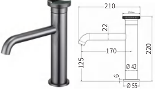
TX22042-Q 铜面盆龙头（枪灰） Brass basin mixer (Gunmetal) 单位 Unit: mm
