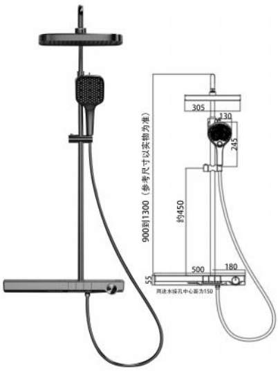
MZH940500-Q 恒温配套（枪灰） Temperature control set (Gunmetal) 淋浴、手持 Shower, hand
