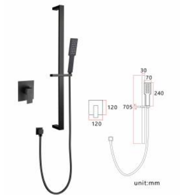
12T1S-H 单功能调温配套（黑色） Single function temperature control set (Black) 手持 Hand 单位 Unit: mm
