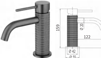
TX15942-Q 铜面盆龙头（枪灰） Brass basin mixer (Gunmetal) 单位 Unit: mm
