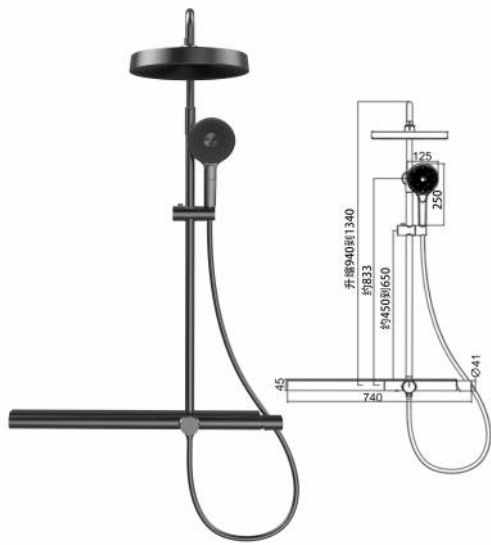
MZ940740-Q 调温配套（枪灰） Thermoregulation control set (Gunmetal) 淋浴、手持 Shower, hand
