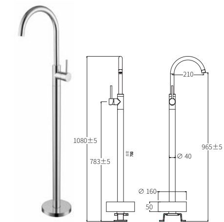
LDR003 明装装落地浴缸龙头（铬色） Floor-to-ceiling bathtub mixer (Chrome)
