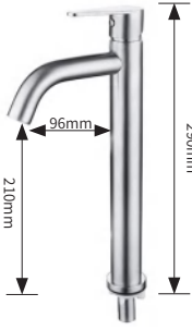
TXDL17530-S 304 不锈钢面盆单冷龙头（拉丝） 304 stainless steel basin mixer (Brushed) 单位 Unit: mm
