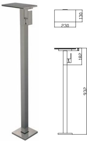
LZ05Y-Q 明装落地浴缸龙头（枪灰） Floor-to-ceiling bathtub mixer (Gunmetal)
