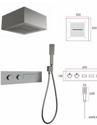
14AH3S142-Q 3 功能恒温套装（枪灰） Three -features thermostatic set (Gunmetal) 雨淋、瀑布、手持 Rain shower, waterfall, hand 单位 Unit： mm
