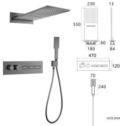
14AH3S092-Q 3 功能恒温套装（枪灰） Three -features thermostatic set (Gunmetal) 瀑布、雨淋、手持 Waterfall, rain, hand 单位 Unit: mm
