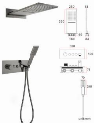
05AH3+1S092-Q 3 功能恒温套装（枪灰） Three-function thermostatic set (Gunmetal) 瀑布、雨淋、手持 Waterfall, rain, hand 单位 Unit: mm
