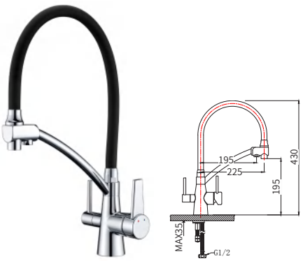
TCP43042-3 铜厨房抽拉龙头（镀铬） Brass pull out kitchen mixer (Chrome) 单位 Unit: mm
