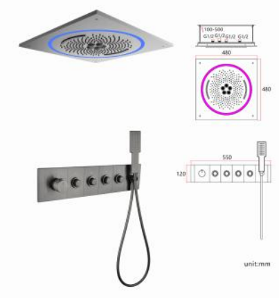
13AH4+1B193L-Q 4 功能 LED 恒温套装（枪灰） Four -features LED thermostatic set (Gunmetal) 雨淋、双瀑布、气泡、手持 Rain shower, double waterfall, bubble, hand 单位 Unit: mm
