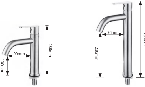
TXDL17530-S 304 不锈钢面盆单冷龙头（拉丝） 304 stainless steel basin mixer (Brushed) 单位 Unit: mm
