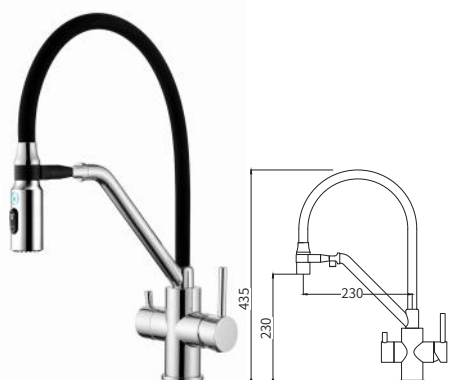
TCP43542-3 铜多功能厨房龙头（镀铬） Brass multi-functional kitchen mixer (Chrome) 单位 Unit: mm
