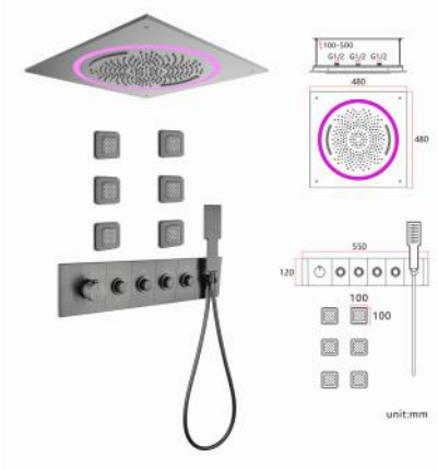
13AH4+1B192LJ4-Q 4 功能 LED 恒温套装（枪灰） Four -features LED thermostatic set (Gunmetal) 雨淋、双瀑布、背喷、手持 Rain shower, double waterfall, back spray, hand 单位 Unit: mm
