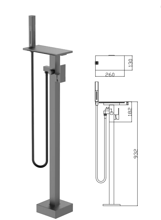
LD05Y2-Q 明装落地浴缸瀑布（枪灰） Floor-to-ceiling bathtub waterfall (Gunmetal)
