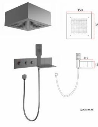
13AH2S141-Q 2 功能恒温套装（枪灰） Two -features thermostatic set (Gunmetal) 雨淋、手持、置物架 Rain shower, handheld, shelving 单位 Unit： mm
