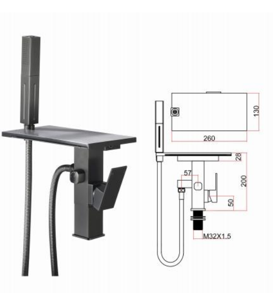
TM05Y2-Q 2 功能台面浴缸瀑布（枪灰） 2 Feature countertop bathtub waterfall (Gunmetal)
