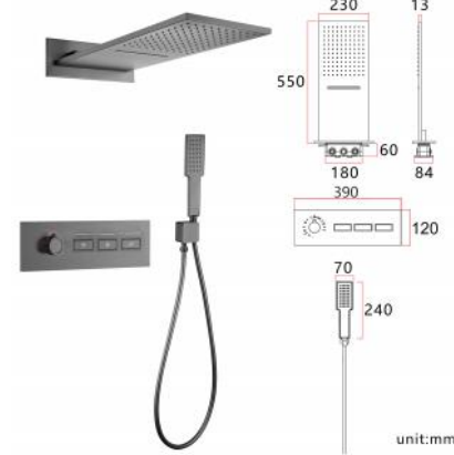
09AH3S092-Q 3 功能恒温套装（枪灰） Three -features thermostatic set (Gunmetal) 瀑布、雨淋、手持 Waterfall, rain, hand 单位 Unit: mm
