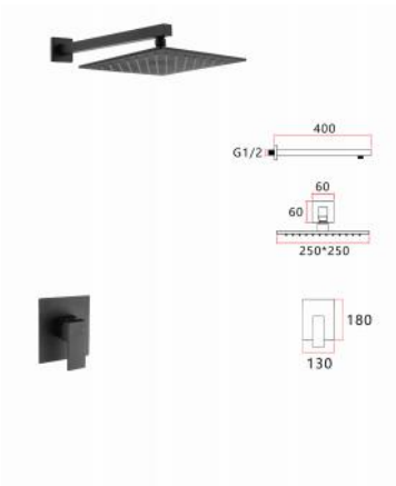
13T1B10-H 单功能调温配套（黑色） Single function temperature control set (Black) 淋浴 Shower 单位 Unit: mm
