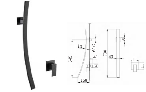
3T1Y02-H 调温入墙龙头（黑色） Thermostat tap into wall (Black) 单位 Unit: mm
