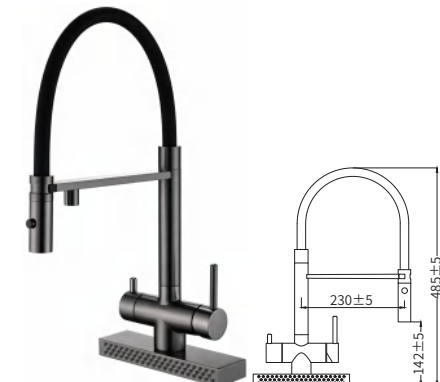
TCP48543-4Q 铜厨房抽拉龙头（枪灰） Brass pull out kitchen mixer (Gunmetal) 单位 Unit: mm
