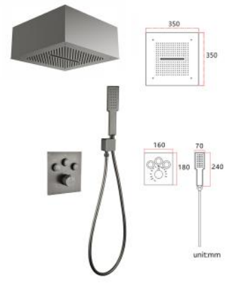
16AH3S142-Q 3 功能恒温套装（枪灰） Three -features thermostatic set (Gunmetal) 雨淋、瀑布、手持 Rain shower, waterfall, hand 单位 Unit： mm
