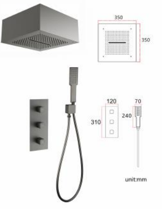
99T3S142-Q 3 功能调温套装（枪灰） Three -features thermoregulation set (Gunmetal) 雨淋、瀑布、手持 Rain shower, waterfall, hand 单位 Unit： mm
